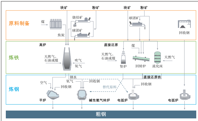
图1：炼钢工艺
