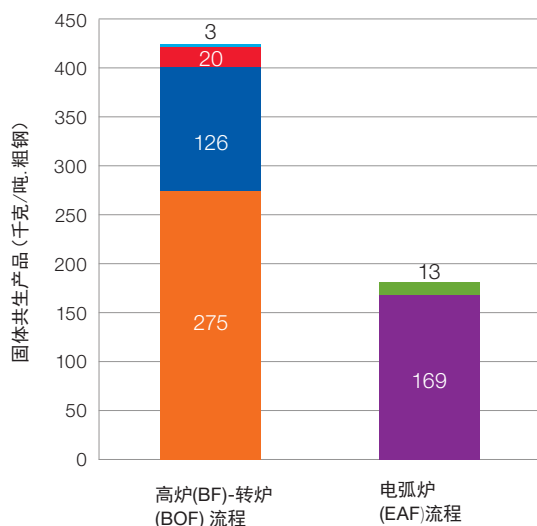
两种钢铁生产流程的主要固体共生产品 1 (平均产量 千克/吨 粗钢)
