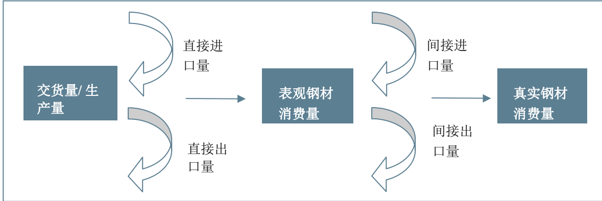
图 2：钢材间接贸易概念
