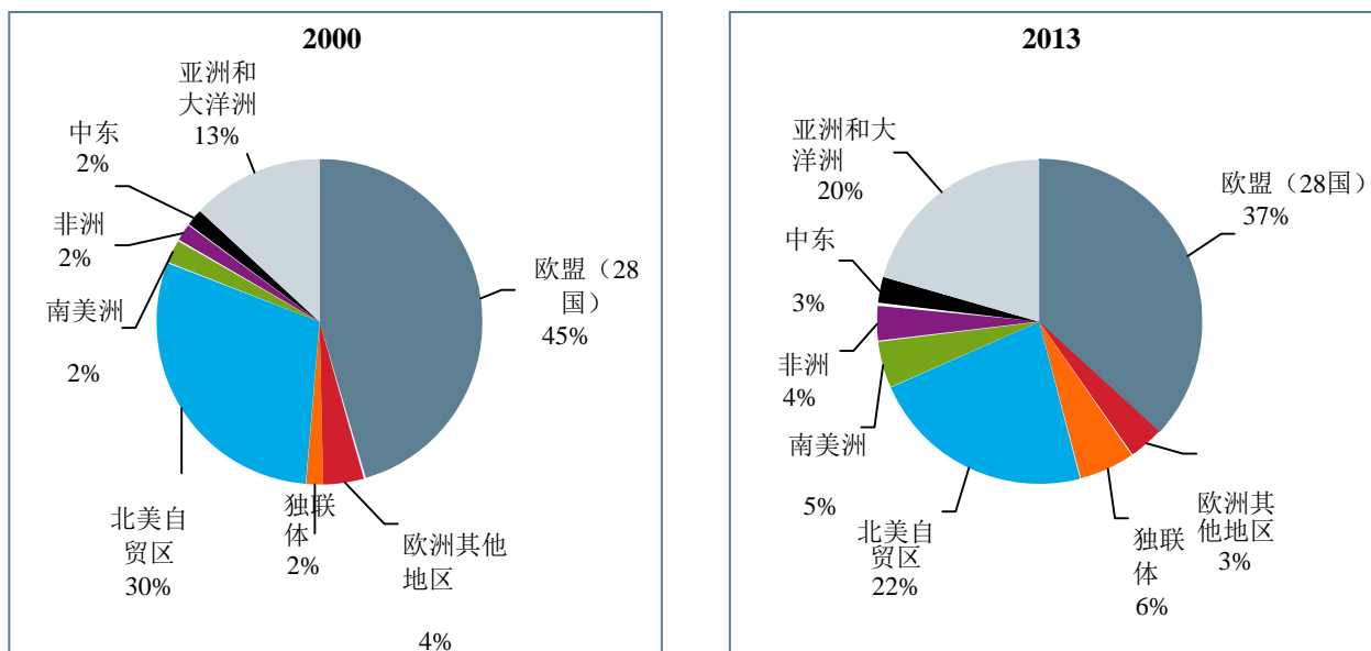
图 6：2000 年和 2013 年钢材间接进口量各地区所占比例
