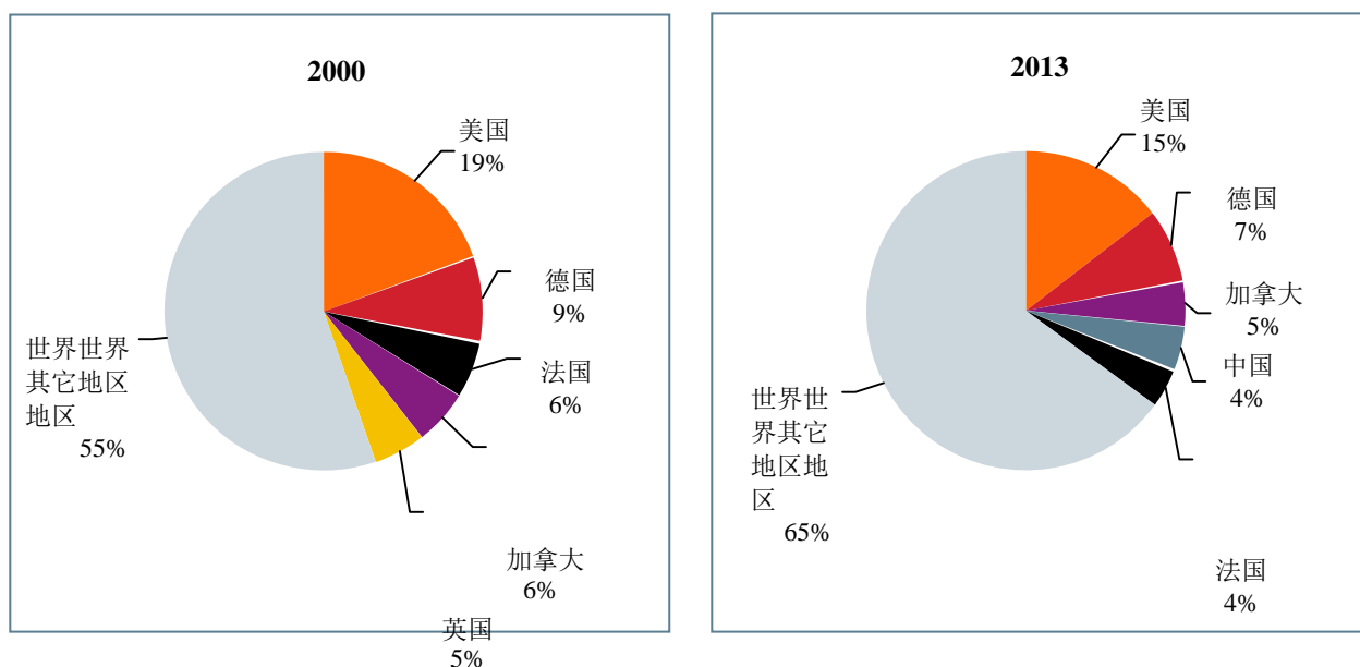
图9：2000年和2013年世界五大进口国在钢材间接进口量中所占比例
