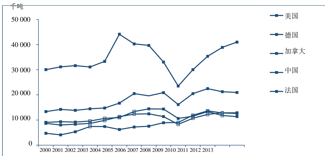
图10：2000-2013年间5大钢材进口国的钢材间接进口量，千吨 (kt)，等值成品钢材
