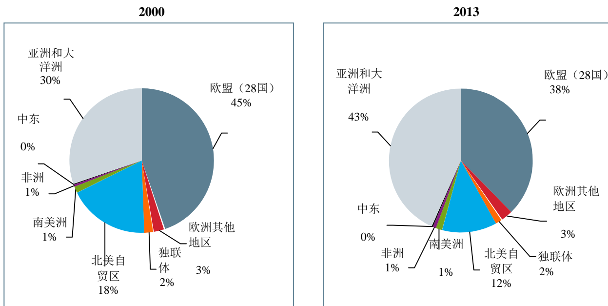
图 5：2000 年和 2013 年钢材间接出口量各地区所占比例
