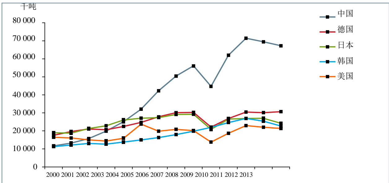
图8：2000-2013年间5大钢材出口国的钢材间接出口量，千吨 (kt)，等值成品钢材
