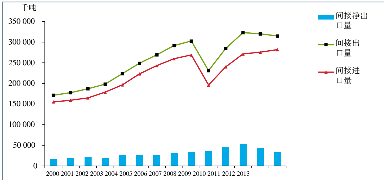
图 4：2000-2013 年间钢材间接出口量、进口量和净出口量，千吨 (kt)，等值成品钢材 来源：国际钢铁协会
