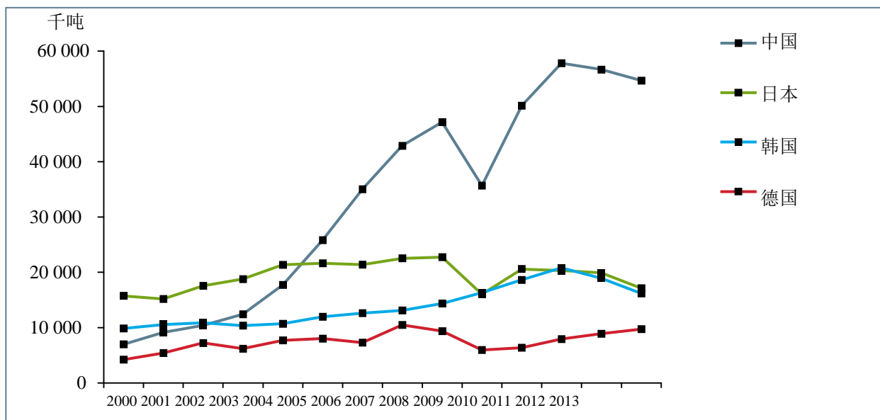
图 11: 2000-2013 年间所选净出口国的钢材间接净出口量, 千吨, 等值成品钢材 来源: 国际钢铁协会
