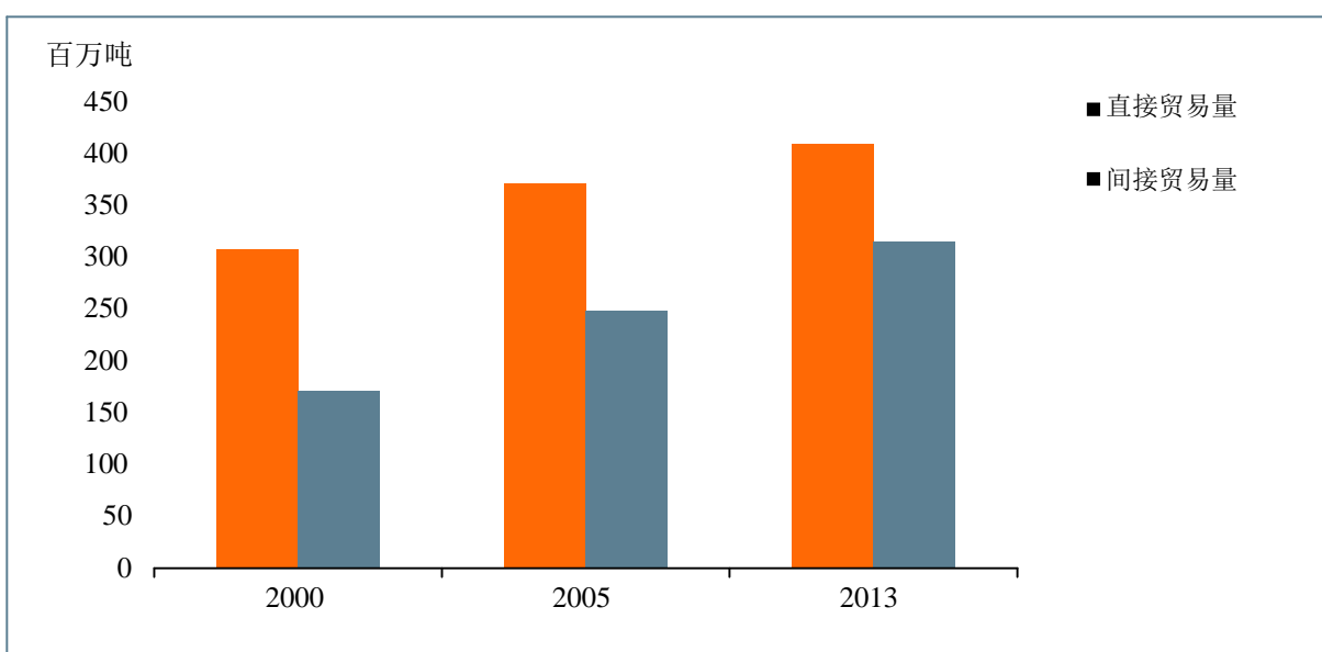
图 1：2000、2005 和 2013 年的世界钢材的直接和间接贸易量 1
