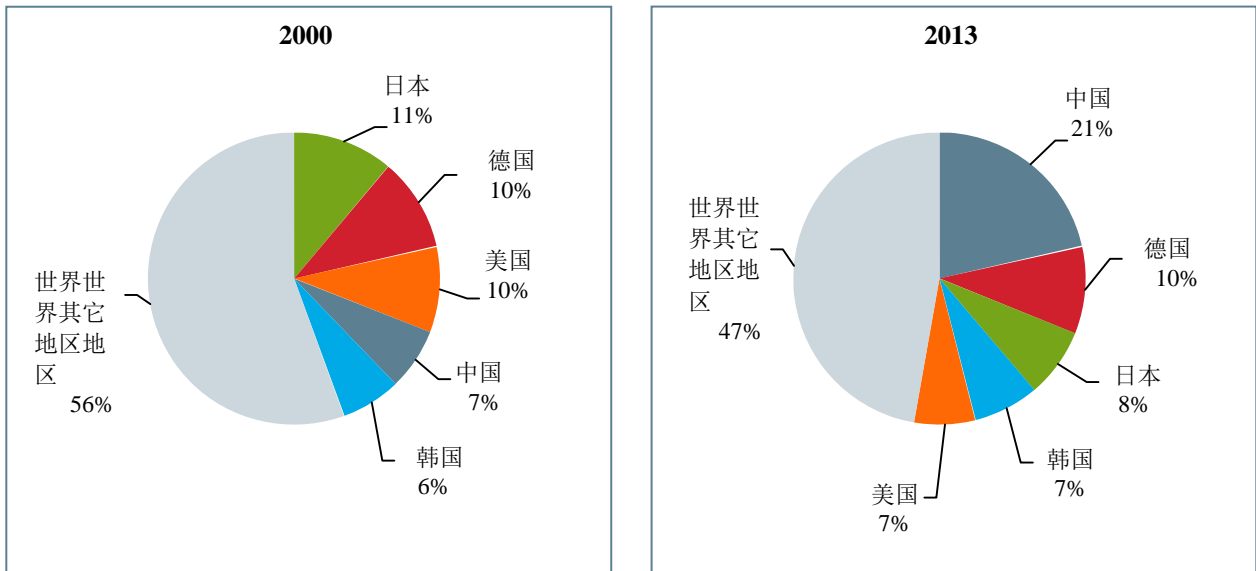
图7：2000年和2013年世界五大出口国在钢材间接出口量中所占比例
