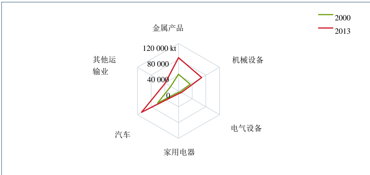
图 13：2003 和 2013 年各行业钢材间接出口量，千吨，等值成品钢材
