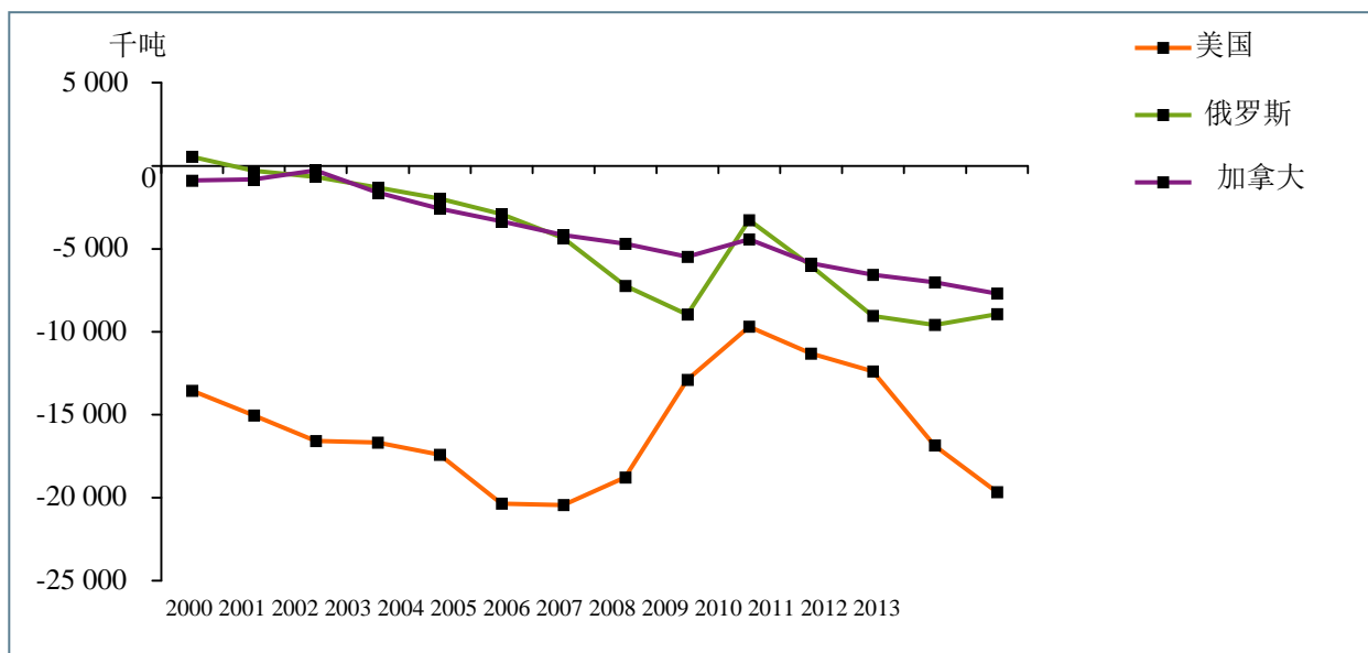
图 12: 2000-2013 年间所选净进口国的钢材间接净出口量, 千吨, 等值成品钢材 来源: 国际钢铁协会
